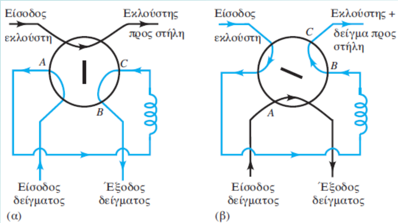
Περιστροφική βαλβίδα δείγματος: (α) θέση πλήρωσης του βρόχου δείγματος ACB , (β) εισαγωγή του δείγματος στη στήλη.
