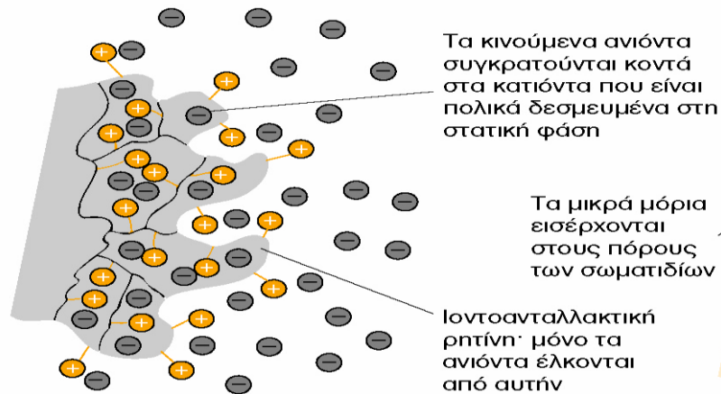
Χρωματογραφία ιοντοανταλλαγής
