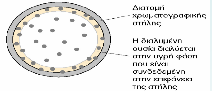
Χρωματογραφία κατανομής
