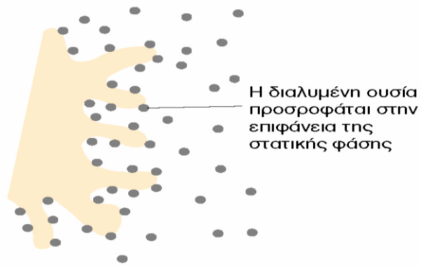
Χρωματογραφία προσρόφησης
