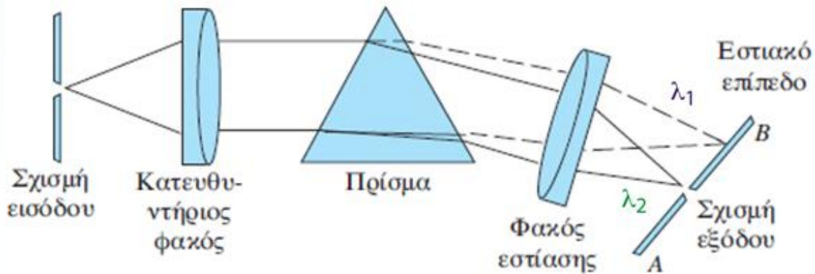
πρίσμα Bunsen
