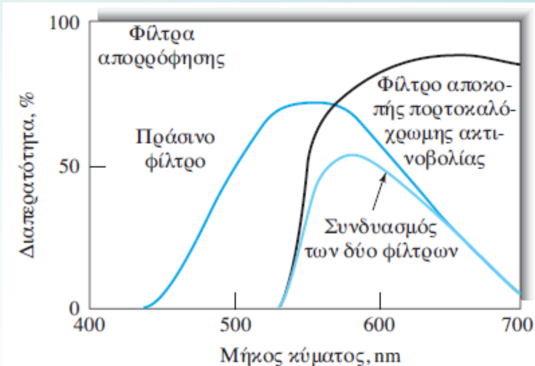
Σύγκριση διάφορων τύπων φίλτρων ορατής ακτινοβολίας
