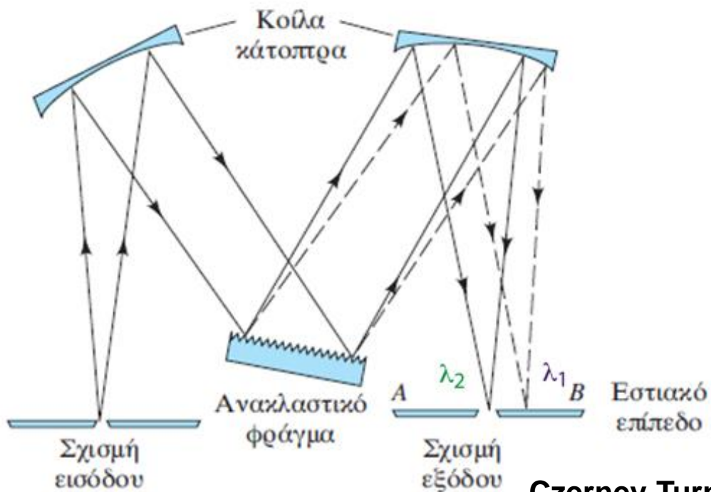
Κοίλα κάτοπτρα Ανακλαστικό φράγμα Σχισμή εισόδου Σχισμή εξόδου Εστιακό επίπεδο Czerny-Turner
