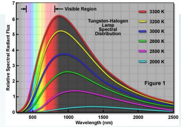
Φάσμα λυχνίας βολφραμίου (πυράκτωσης)
