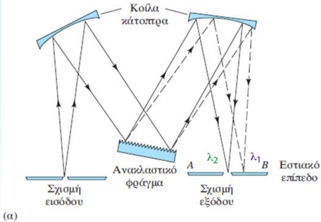
Czerney-Turner
