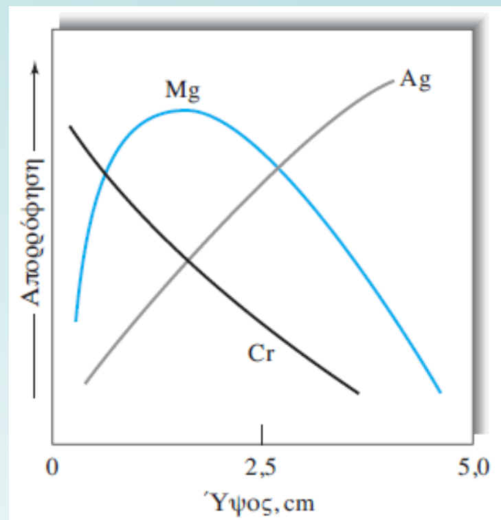
Κατατομή απορρόφησης από τη βάση της φλόγας-καυστήρα για τρία στοιχεία.
