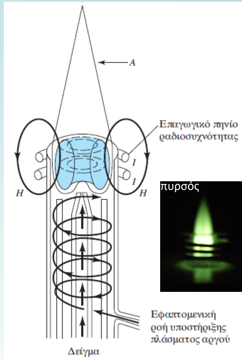
Τυπική πηγή επαγωγικά συζευγμένου πλάσματος.
