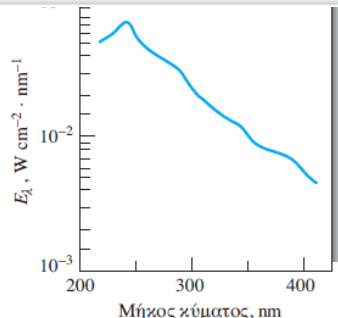
Φάσμα λυχνίας δευτερίου
