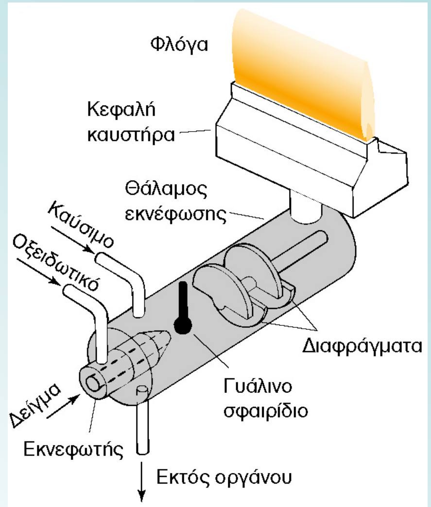
Καυστήρας νηματικής ροής.
