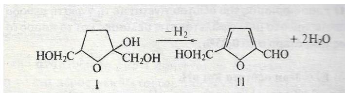
Σχήμα. Σχηματισμός υδροξυμεθυλοφουρφουράλης (II) από την φρουκτόζη (I).
