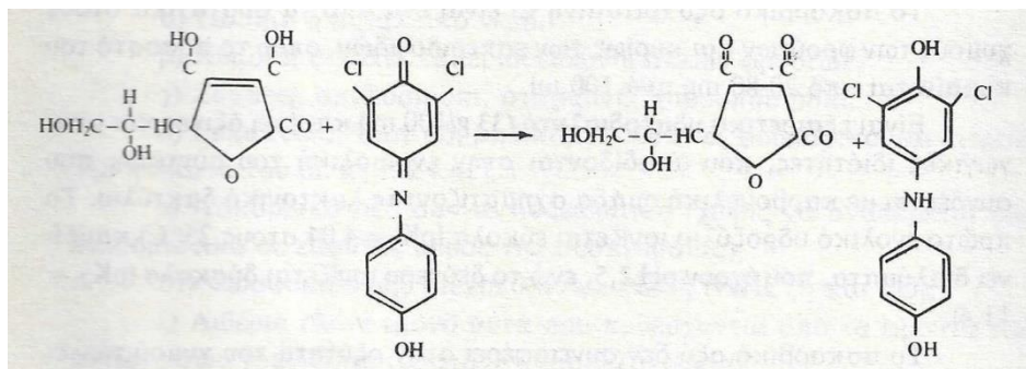
Σχήμα. Οξείδωση του ασκορβικού οξέος από την 2,6-διχλωροφαινολινδοφαινόλη.
