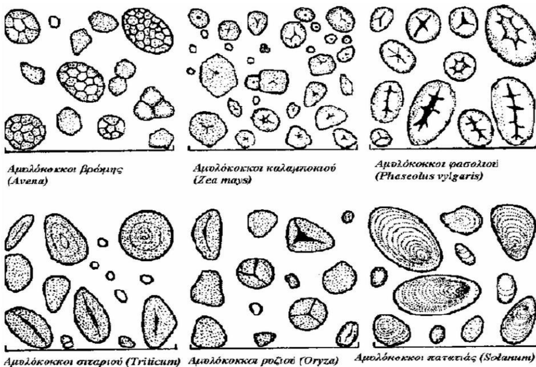
Σχήμα. Εικόνες από μικροσκόπιο κόκκων αμύλου από διάφορες πηγές.
